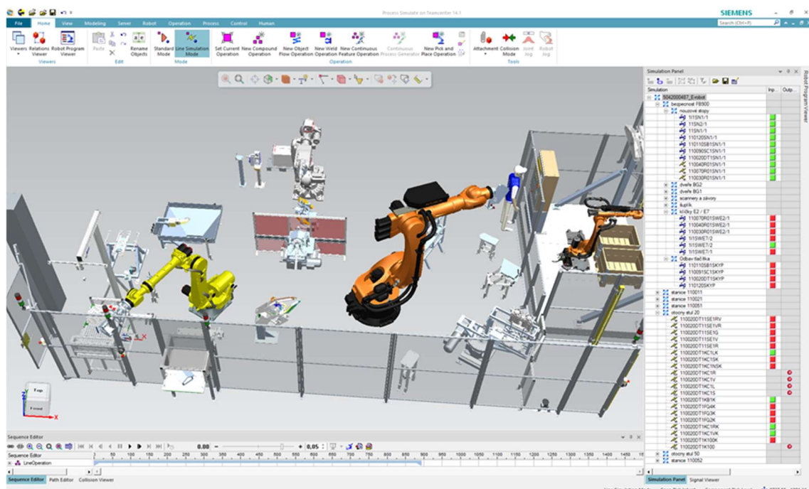
Obr.2: Robotické pracoviště v prostředí Process Simulate + Virtuální Zprovoznění (signály: nouzové stopy, odbav. tlačítka, přípravky atd.).
